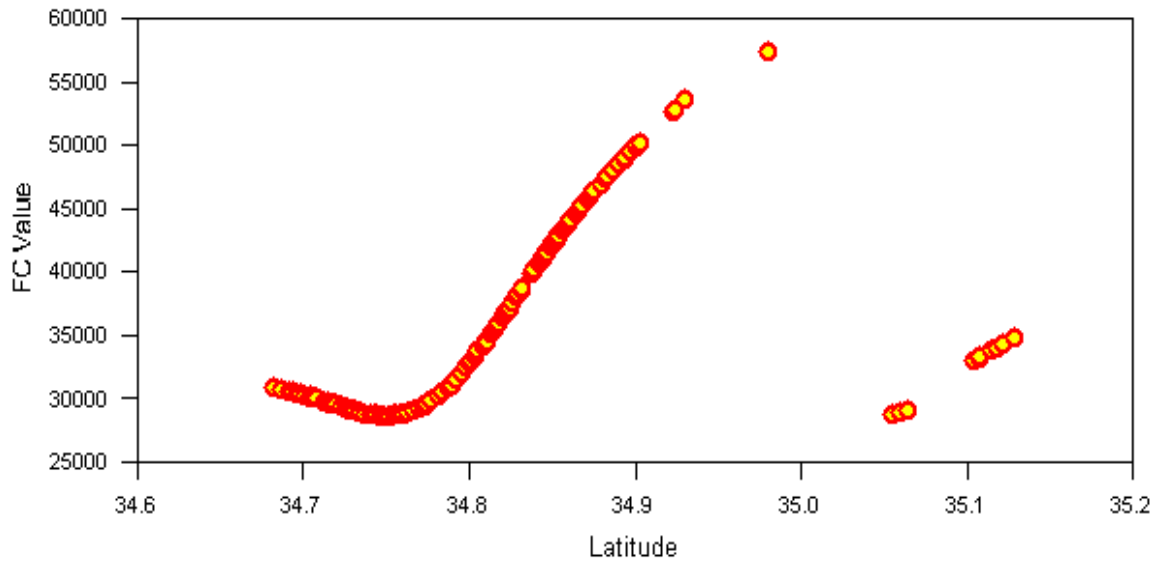
Figure A-13. Influence of Latitude on 30 Year EUR.
